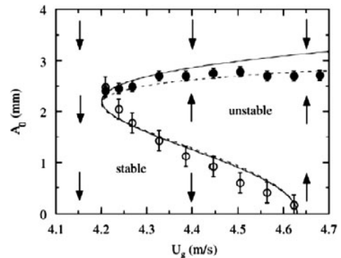
図6 文献[3]より。強制振幅 A_0 とガス速度 U_g （不安定性の駆動力）空間における非線形不安定性のダイアグラムを示す。白丸は亜臨界不安定性の閾値振幅を示す。黒丸は、飽和振幅を示す。曲線は、簡約理論モデルを実験データにフィットして得られたものである。詳細は文献[3]を参照のこと。
